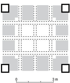
Grundriss Holzturm- fundament
