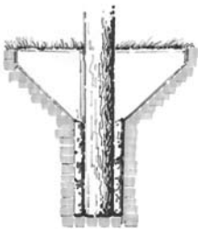
Palisadengraben: Schnitt und Rekonstruktion von WP 10/30
